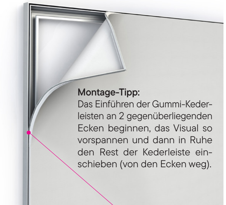
Beispiel Einschub Gummi-Kederleiste in Aluminium-Leiste
